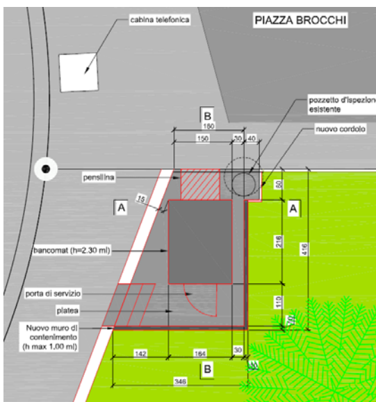
Figura 2: pianta posa "cabina bancomat" Figura 3: fotomontaggio indicativo
